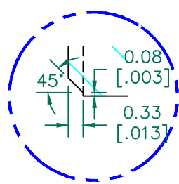
DETAIL "A" SCALE: 6:1
